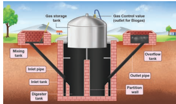
Fig. 9.3 Biogas Unit
